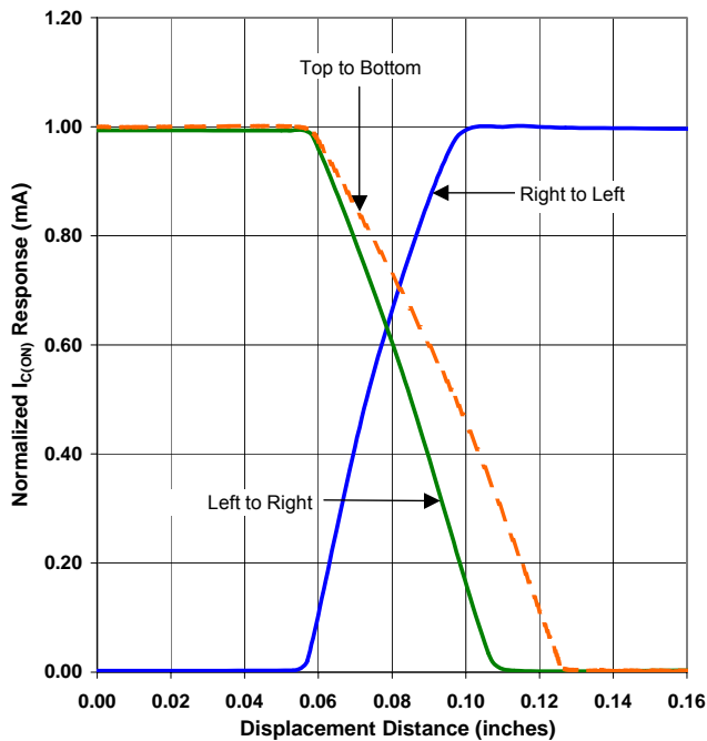
OPB202 - Flag in Middle of Slot
